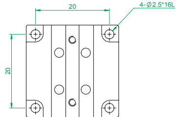
MX(Y)25-A-18系列 底座安裝孔尺寸
