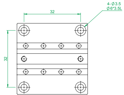
MX(Y)40-A-18系列 底座安裝孔尺寸
