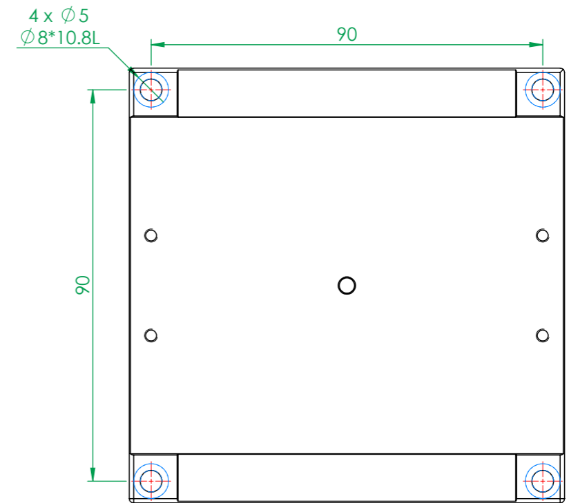
MX(Y)100-S-28系列 底座安裝孔尺寸
