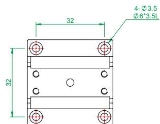
MX(Y)40-S-28系列 底座安裝孔尺寸
