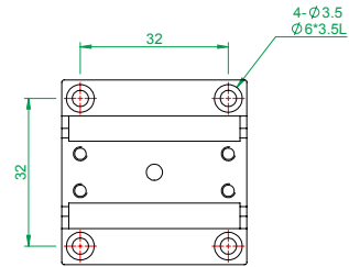
MX(Y)40-S-28系列 底座安裝孔尺寸
