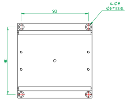
MX(Y)100-S-28系列 底座安裝孔尺寸
