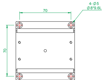
MX(Y)80-S-28系列 底座安裝孔尺寸
