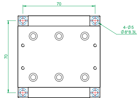
MX(Y)80-A系列 底座安裝孔尺寸
