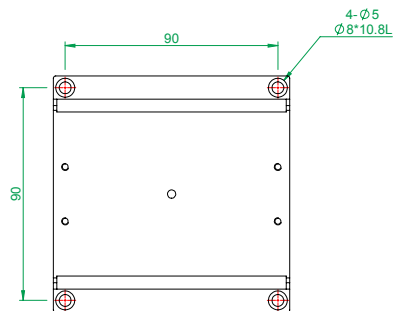
MX(Y)100-S-28系列 底座安裝孔尺寸
