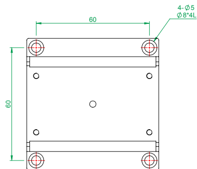
MX(Y)70-S-28系列 底座安裝孔尺寸
