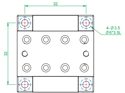
MX(Y)40-A系列 底座安裝孔尺寸
